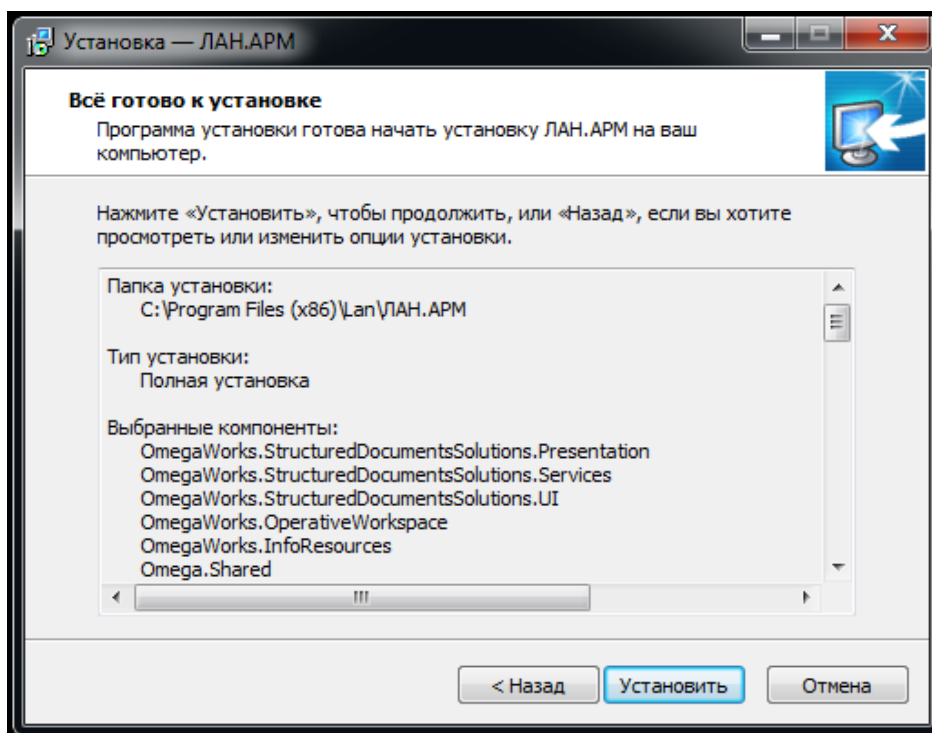
Рисунок 6 – ЛАН.АРМ. Установка
