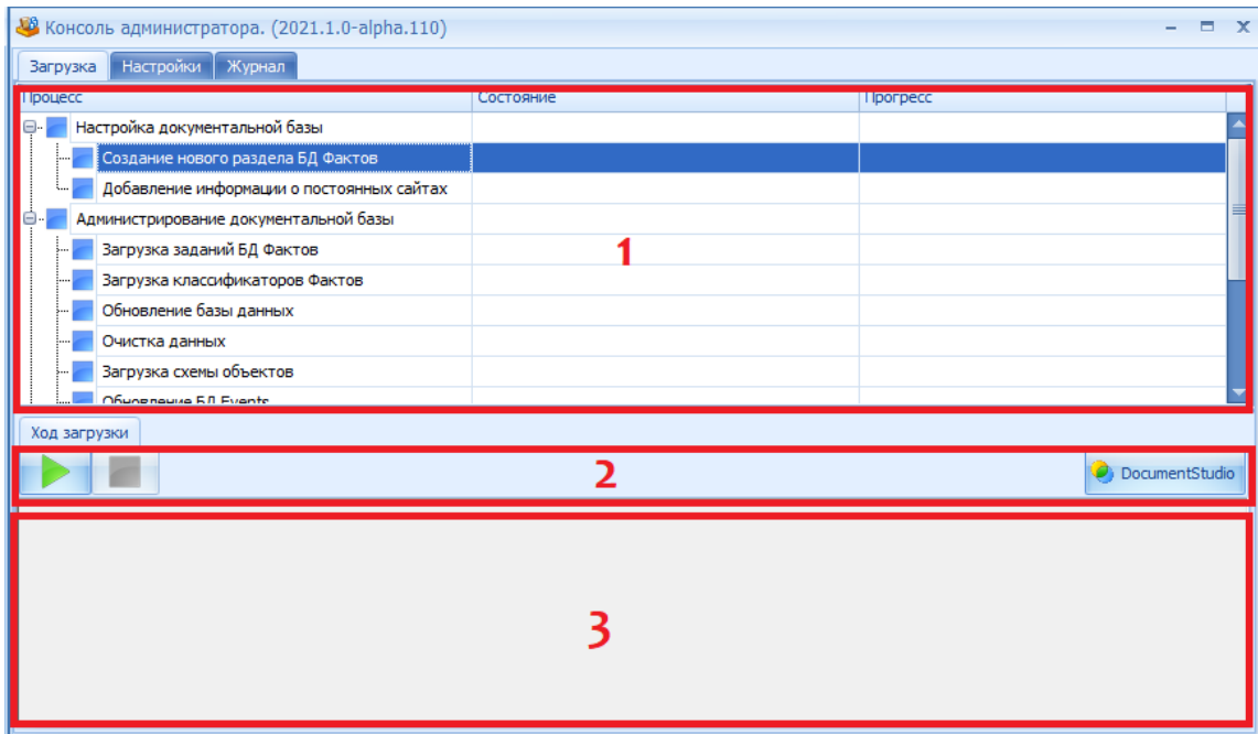
Рисунок 10 – Вкладка «Загрузки»
