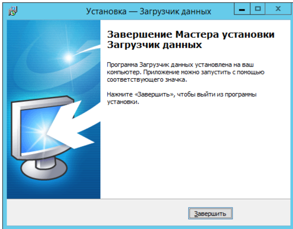
Рисунок 7 – Завершение установки
