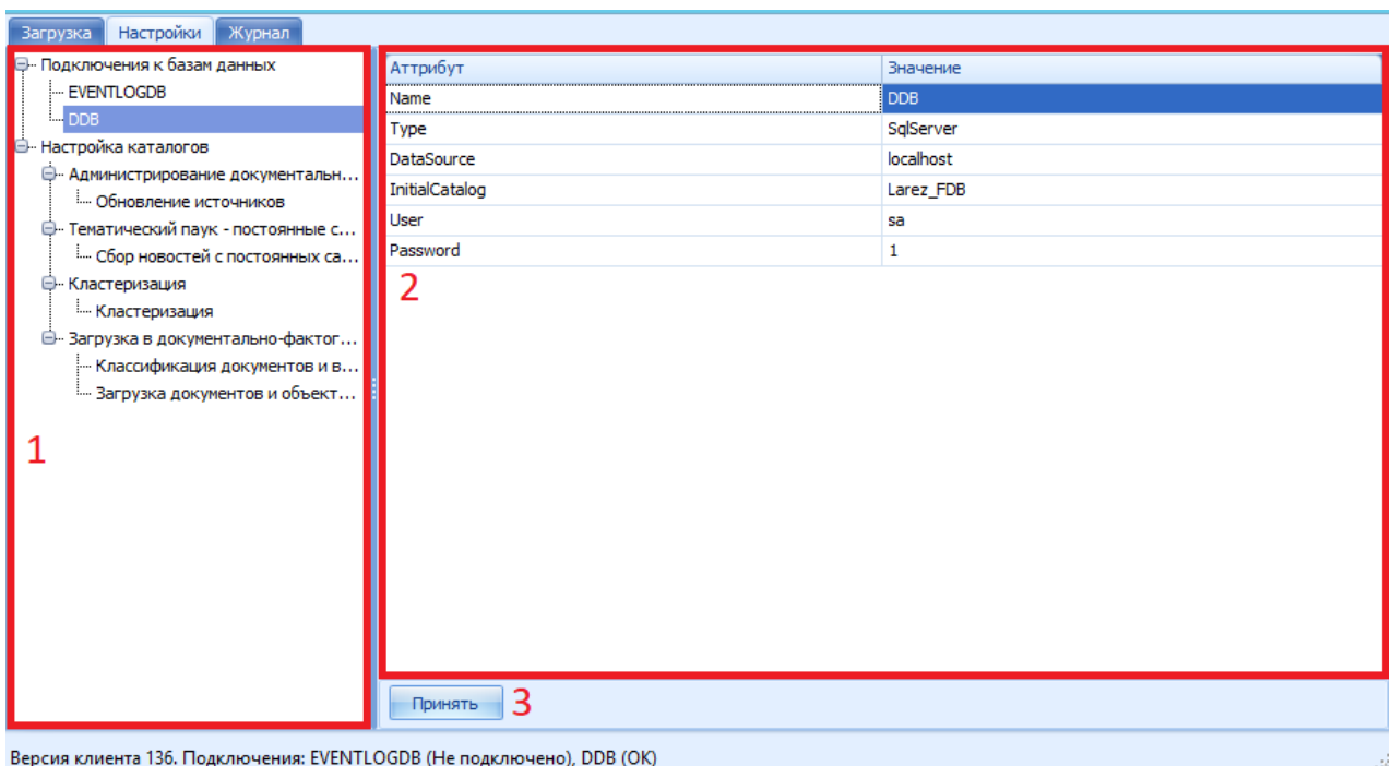
Рисунок 14 – Вкладка «Настройки»
