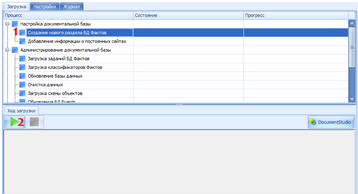
Рисунок 11 – Запуск процесса
